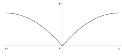
Abbildung 1: f(x) = \frac{|x|}{2} \cdot \left( \pi - \frac{|x|}{2} \right)
