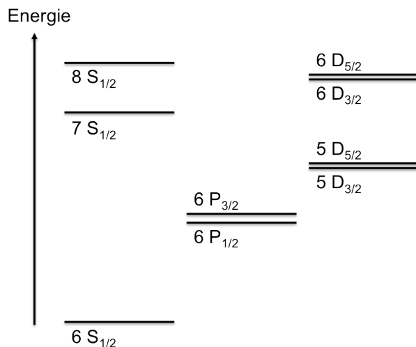
Abbildung 1: Niveauschema von Cäsium mit dem Grundzustand 6S_{1/2} und den ersten angeregten Zuständen.
