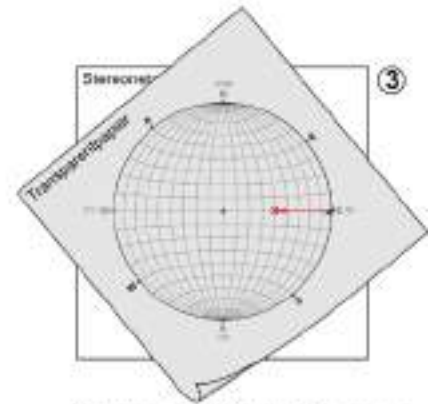
3) Abtragen des 50° Fallwinkels von der Markierung entlang der E-Achse nach innen. (Die Kreuzmarkierung entspricht dem Durchstoßpunkt der Falllinie der Ebene durch die Lagenkugel)
