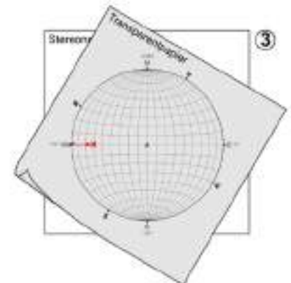
3) Abtragen des 30° Fallwinkels von der Markierung entlang der E-W-Achse nach innen. Die Kreuzmarkierung ist bereits der Durchstoßpunkt des Linears mit der Halbkugel der Projektion!
